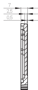
сечение В масштаб 1:1
