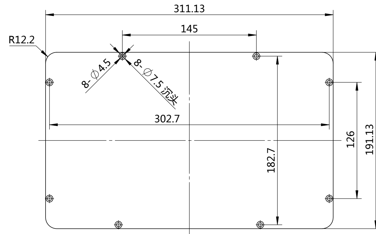
面板尺寸
