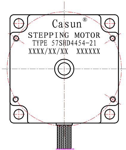
电机规格 Motor specification
