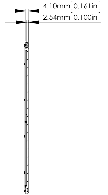
SECTION B-B SCALE 1 : 3
